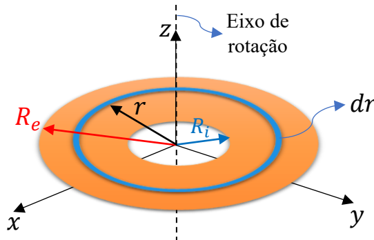
Figura 18 - Elemento infinitesimal de área da coroa circular
