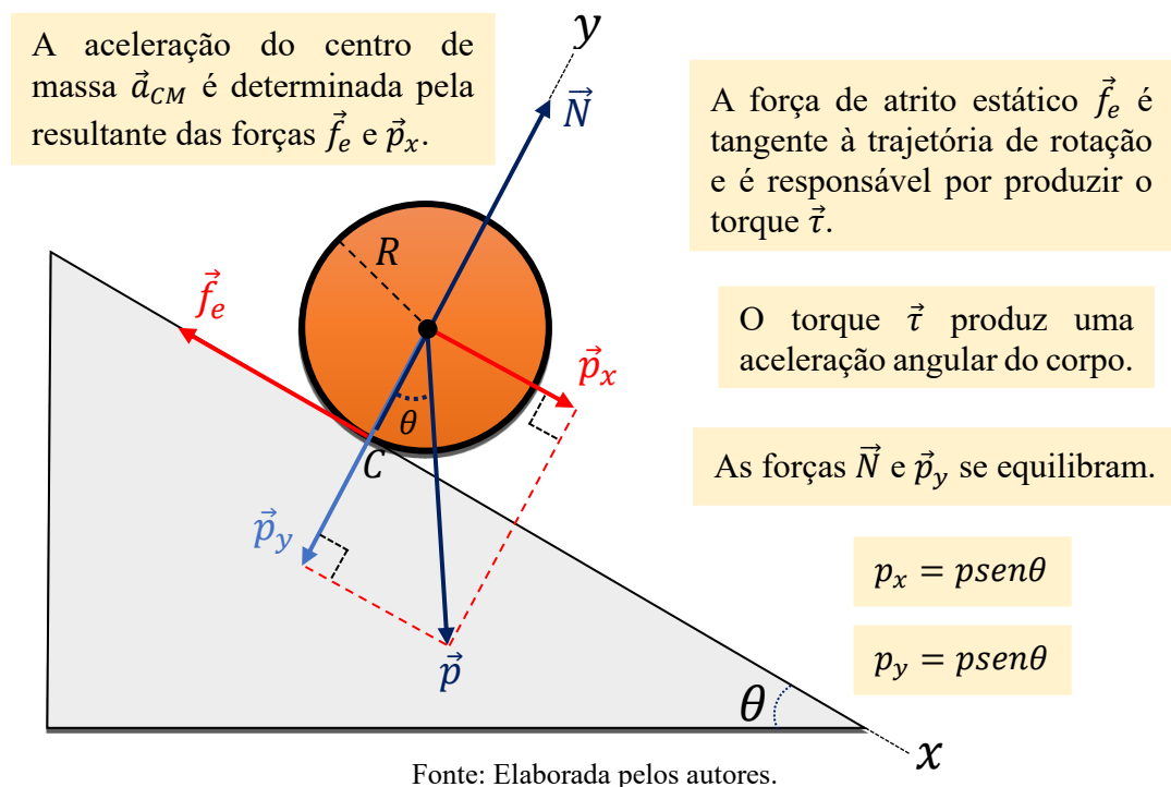
Figura 38 - Corpo redondo em rolamento suave ao longo de um plano inclinado
