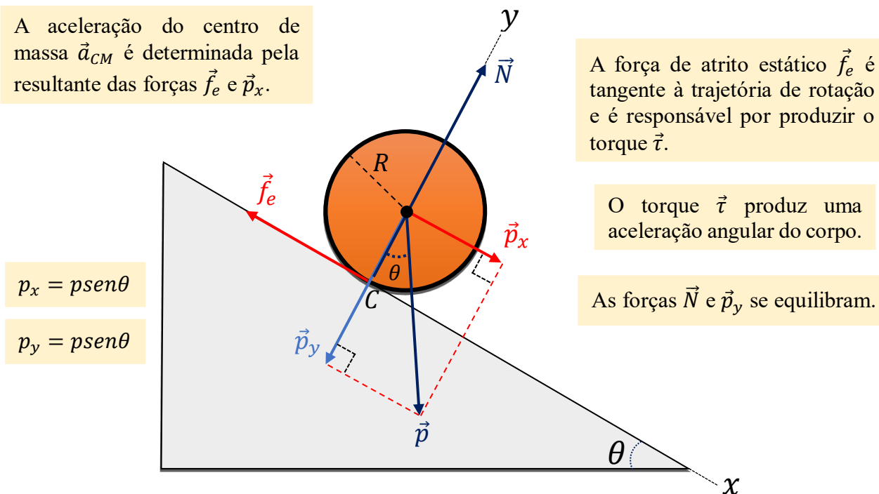
Figura 9.02: Corpo redondo em rolamento suave ao longo de um plano inclinado que forma um ângulo \theta com o plano horizontal.
