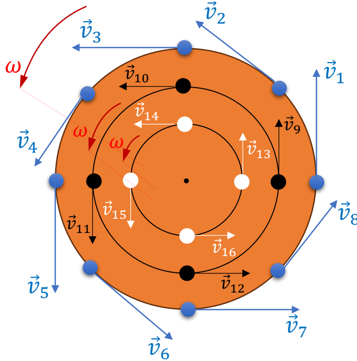
Figura 5 - Corpo rígido circular em rotação em sentido anti-horário, descrevendo um MCU
