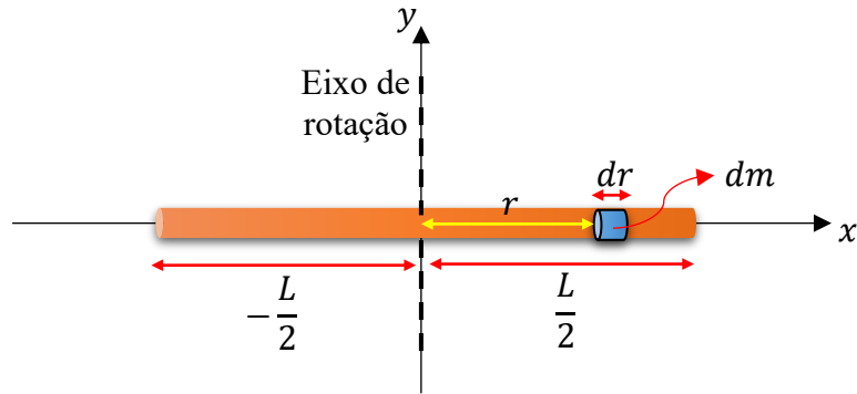
Figura 15 - Barra fina homogênea com eixo central de rotação
