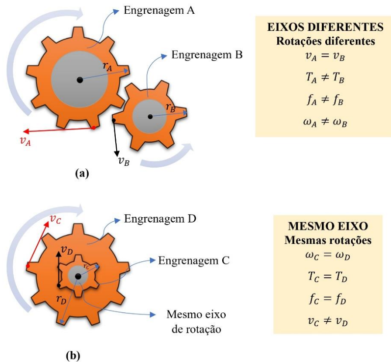
Figura 9 - Transmissão de rotação entre engrenagens
