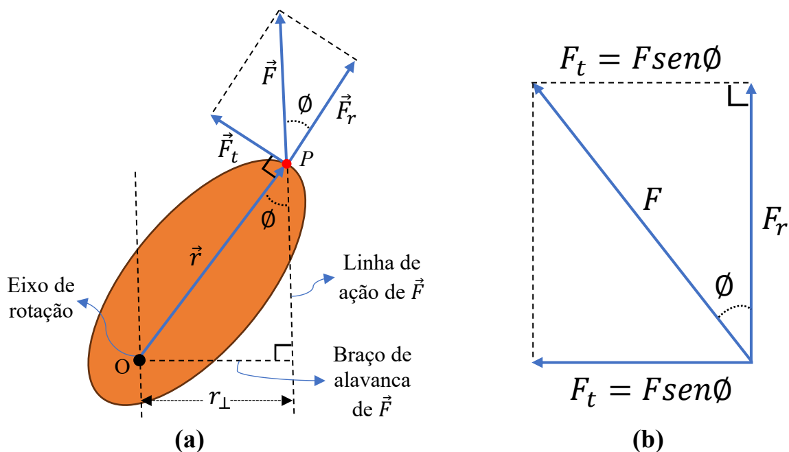
Figura 27 - Corpo rígido sofrendo a ação de uma força \vec{F}
