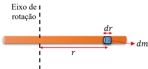
Figura 14 - Elemento infinitesimal de massa dm da barra distante r do eixo de rotação
