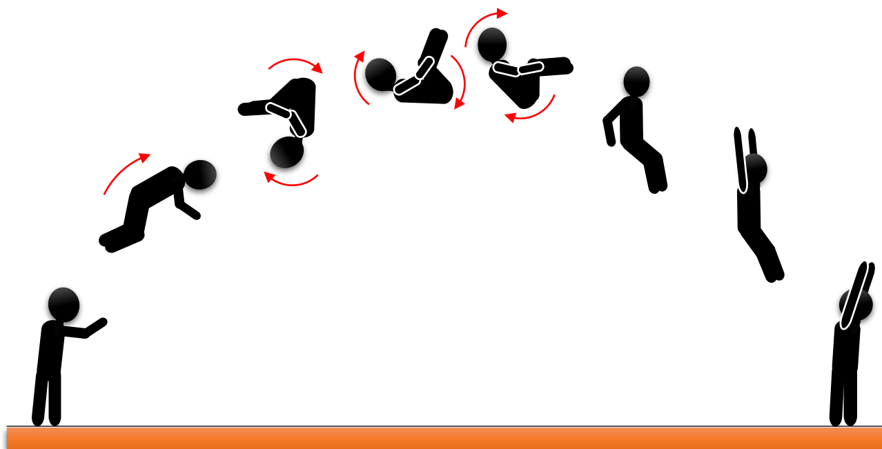
Figura 46 - Representação de um atleta realizando um salto mortal
