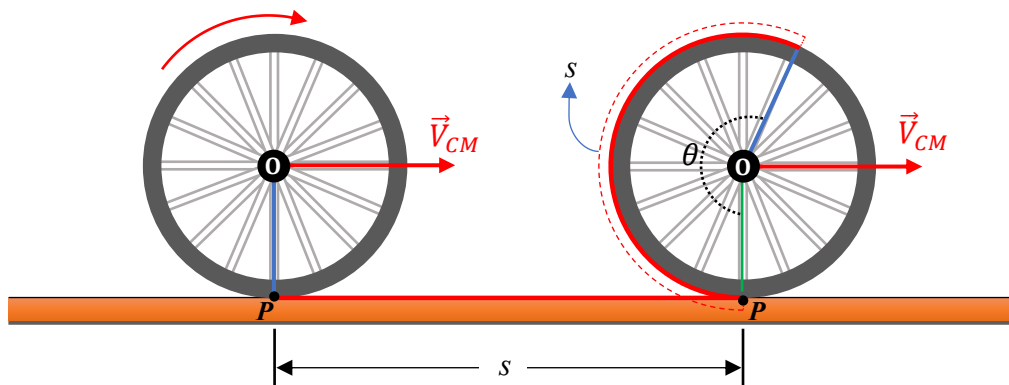
Figura 32 - Roda em rolamento com velocidade do centro de massa \vec{V}_{CM} .
