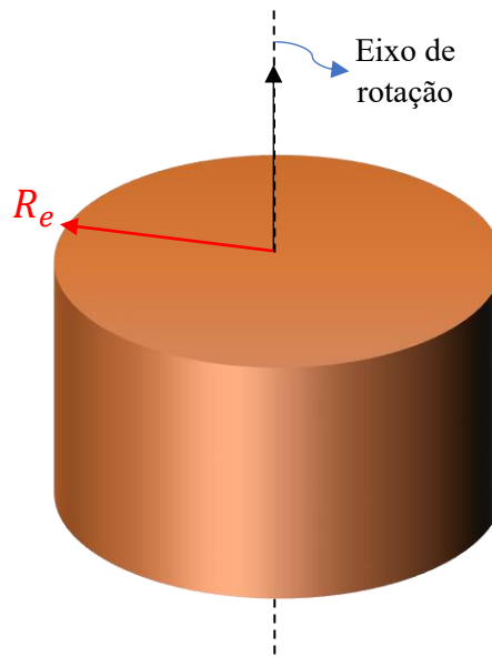
Figura 23 - Cilindro homogêneo de raio R
