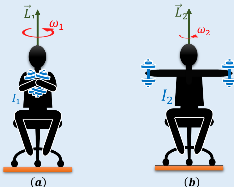
Figura 12.06: Exercício Proposto 12.02 - Representação de um estudante girando em uma cadeira giratória. Em (a), a pessoa está com os braços fechados segurando os halteres enquanto gira. Em (b), a pessoa está com os braços abertos.
