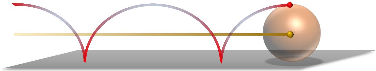
Figura 31 - Esfera maciça homogênea rolando da esquerda para direita sem deslizamento
