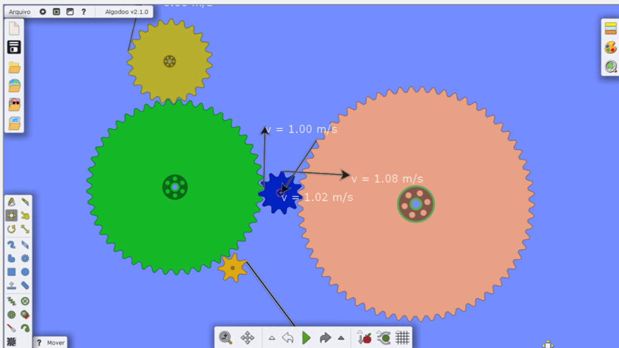
Figura 3.04: Captura de tela do software Algodoo : sistema de engrenagens com contato e com diferentes eixos de rotações. Fonte: os autores.
