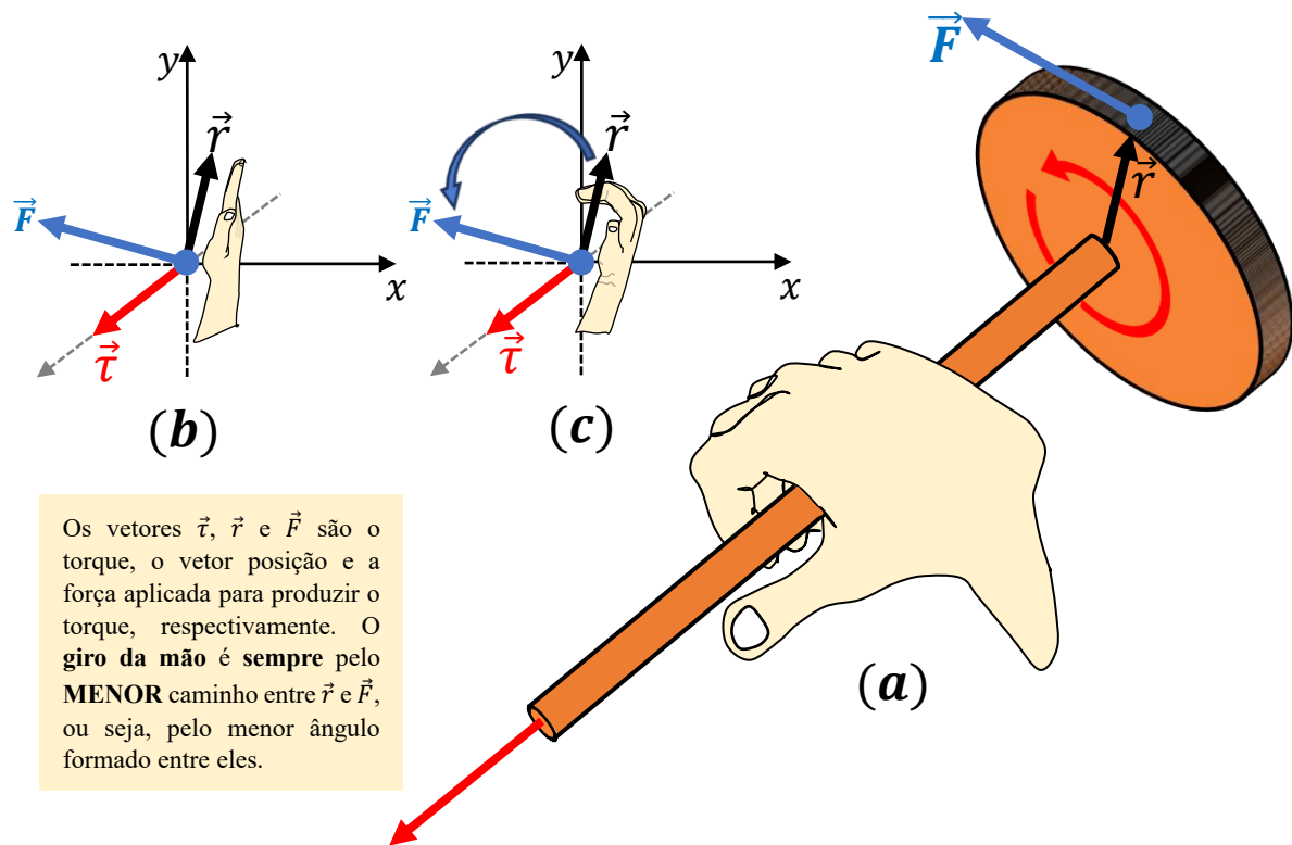
Figura 40 - Regra da mão direita para determinar a orientação do torque
