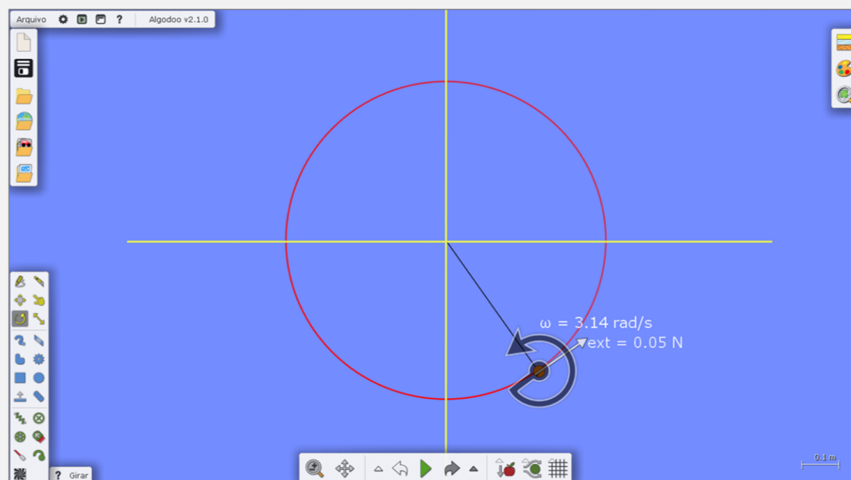
Figura 6.04: Captura de tela do software Algodoo : mesmo corpo de massa m da Figura 6.03 em uma posição angular diferente, preso à extremidade de uma barra fina de massa desprezível, submetido a uma força tangencial de 0,05 N e com velocidade angular de 3,14 rad/s. Fonte: os autores.
