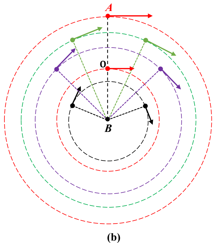
Figura 7.06: Representação do movimento de rolamento como uma rotação pura, com eixo de rotação de passa pelo ponto B. Em (a), a representação dos vetores velocidades em diversos pontos da roda. Em (b), a trajetória circular que esses pontos descreveriam se analisados como rotação pura.
