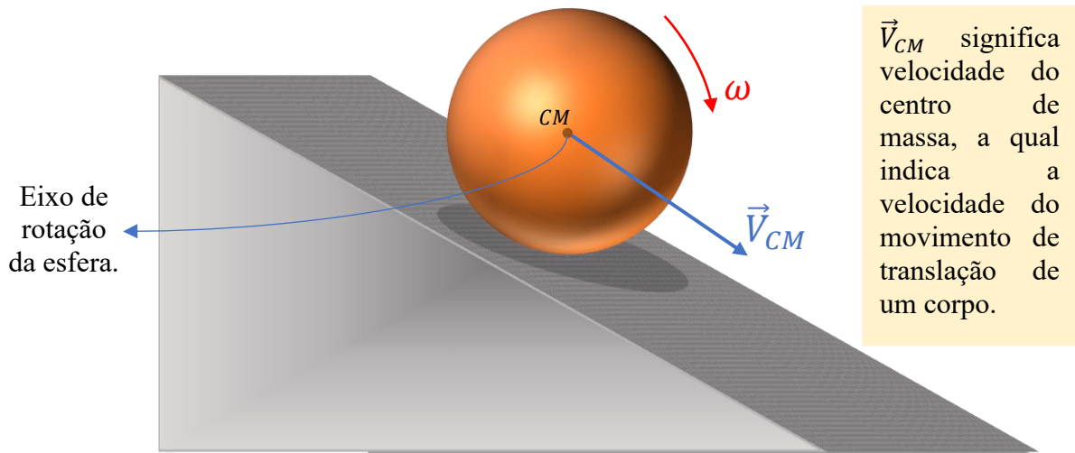
Figura 30 - Esfera homogênea em rolamento sobre um plano inclinado
