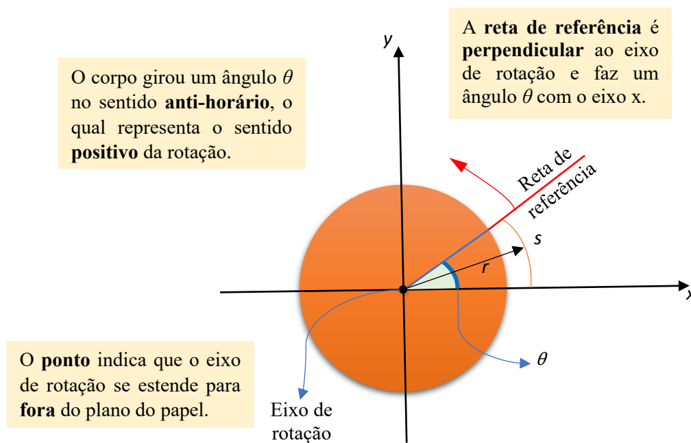
Figura 2 - Disco com rotação em sentido anti-horário
