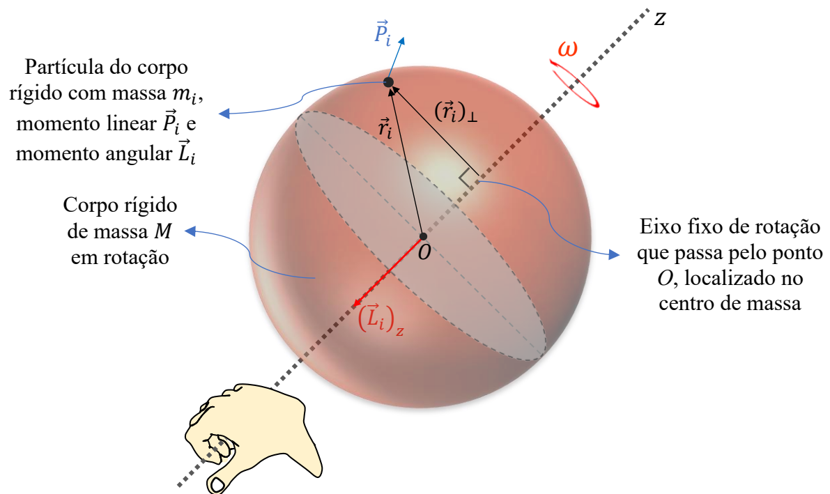
Figura 43 - Esfera homogênea em rotação em relação a um fixo que passa pelo seu CM
