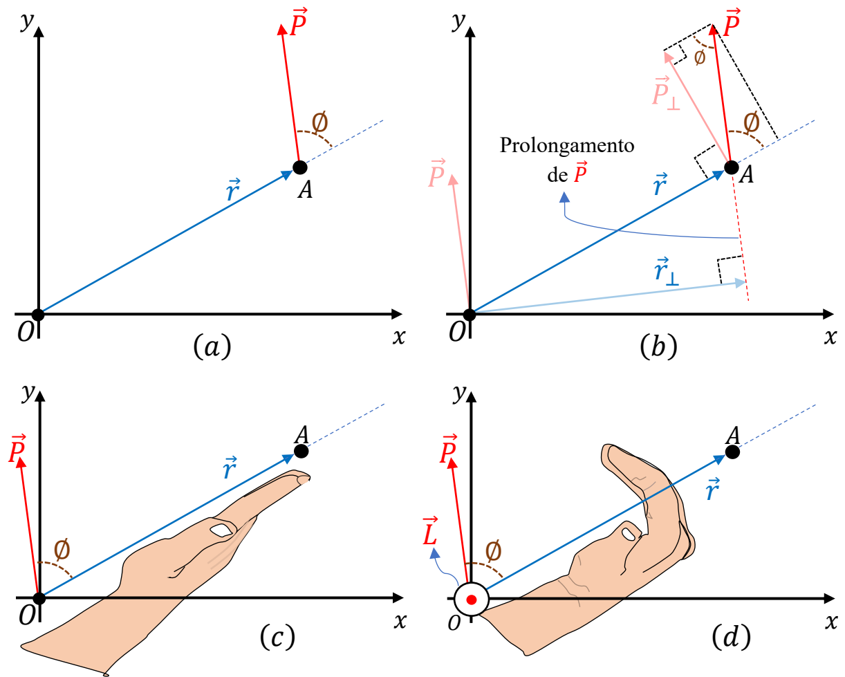
Figura 42 - Regra da mão direita para se obter a orientação do momento angular \vec{L}
