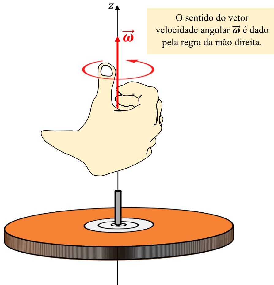
Figura 4 - Sentido do vetor velocidade angular \vec{\omega} de um disco rígido
