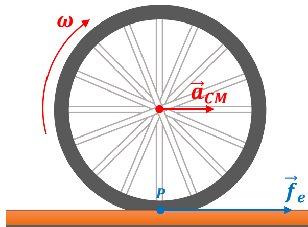
Figura 37 - Roda em movimento acelerado sem sofrer deslizamento
