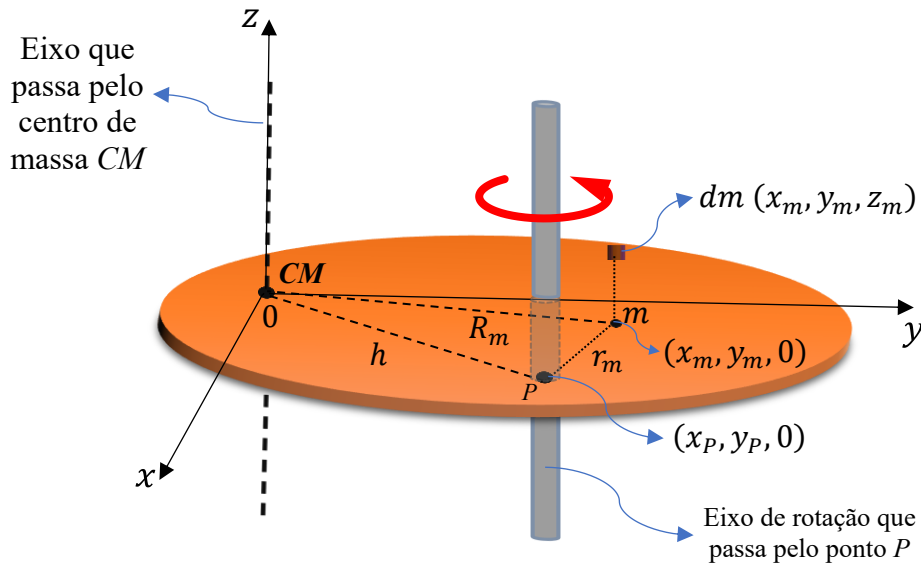
Figura 26 - Eixos paralelos de um corpo rígido
