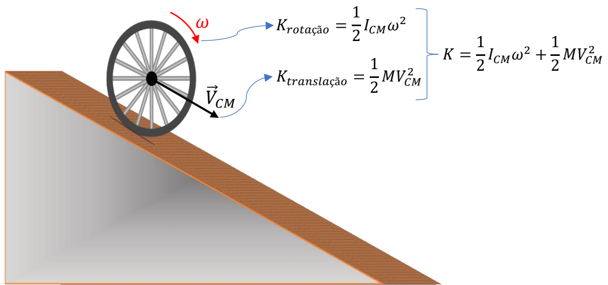
Figura 36 - Roda homogênea em rolamento em um plano inclinado
