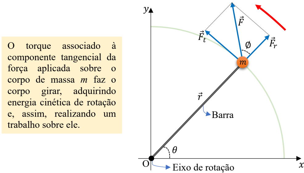
Figura 29 - Corpo rígido de massa m em rotação preso à extremidade de uma barra fina
