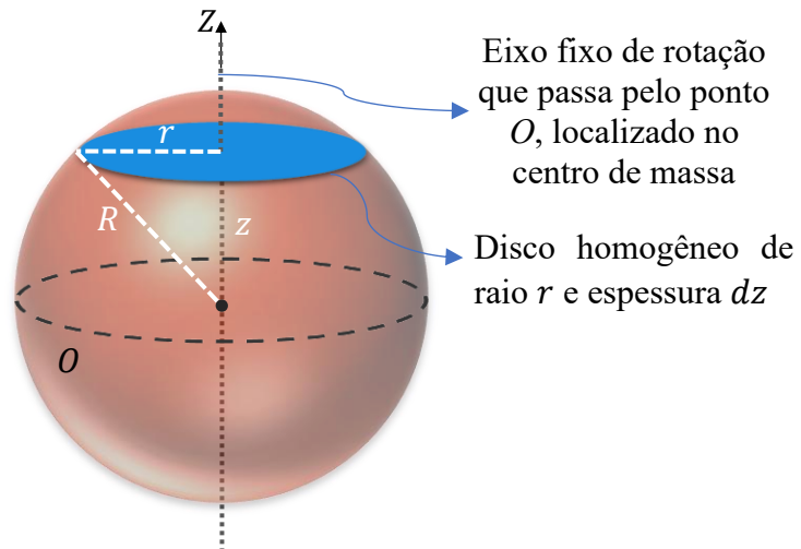
Figura 24 - Esfera homogênea girando em torno de um eixo fixo que passa pelo seu CM
