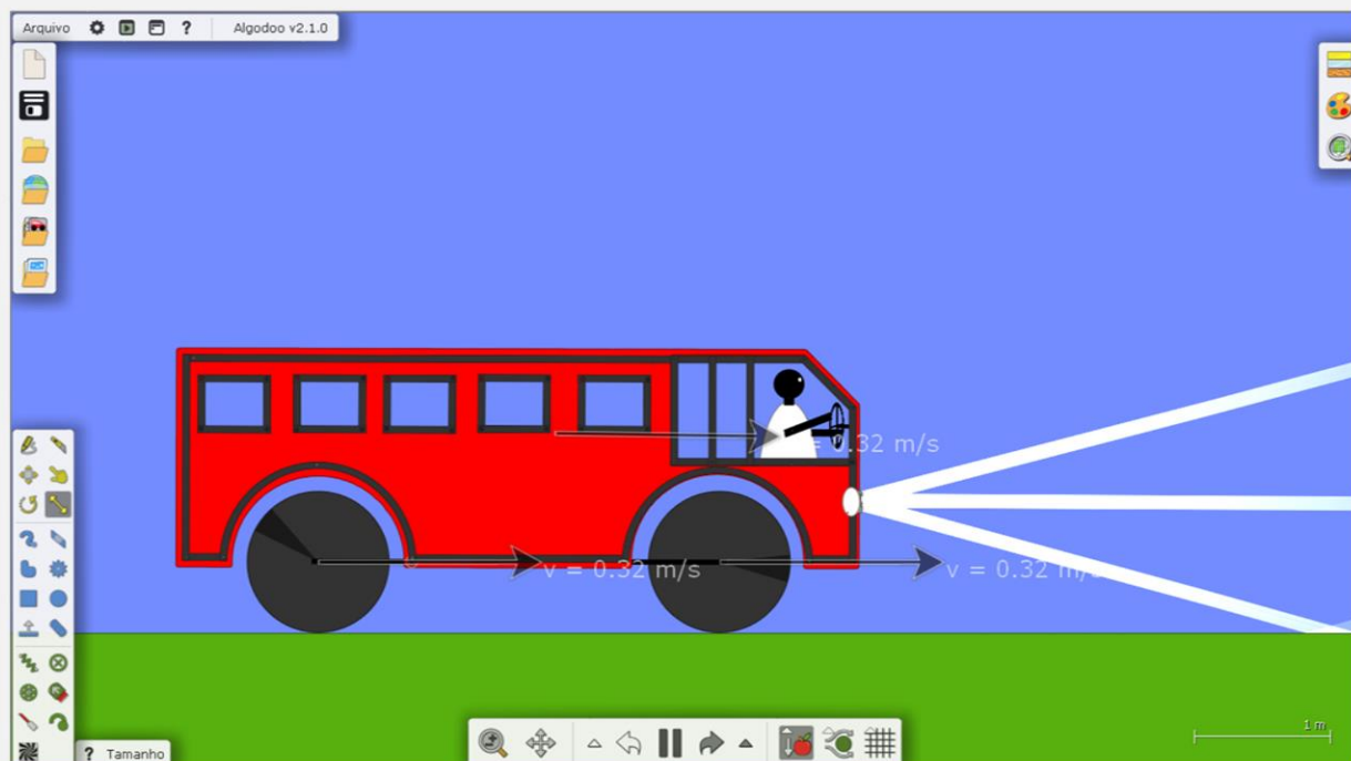
Figura 8.02: Captura de tela do software Algodoo : Ônibus em movimento retilíneo uniforme (MRU) com rodas em movimento de rolagem.
