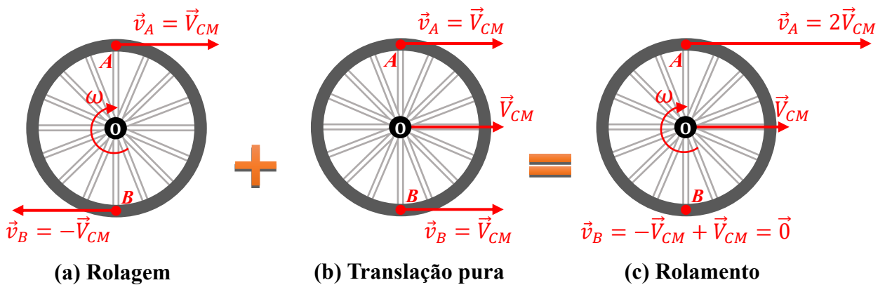
Figura 33 - Combinação dos movimentos de rotação e translação puros de uma roda
