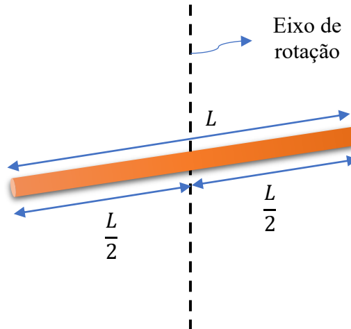
Figura 12 - Barra fina homogênea de comprimento L e eixo central de rotação
