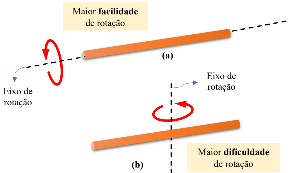
Figura 10- Momentos de inércia diferentes para corpos idênticos
