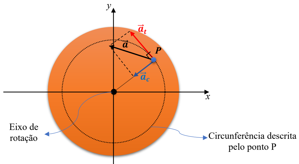
Figura 7 - Corpo rígido em movimento circular acelerado
