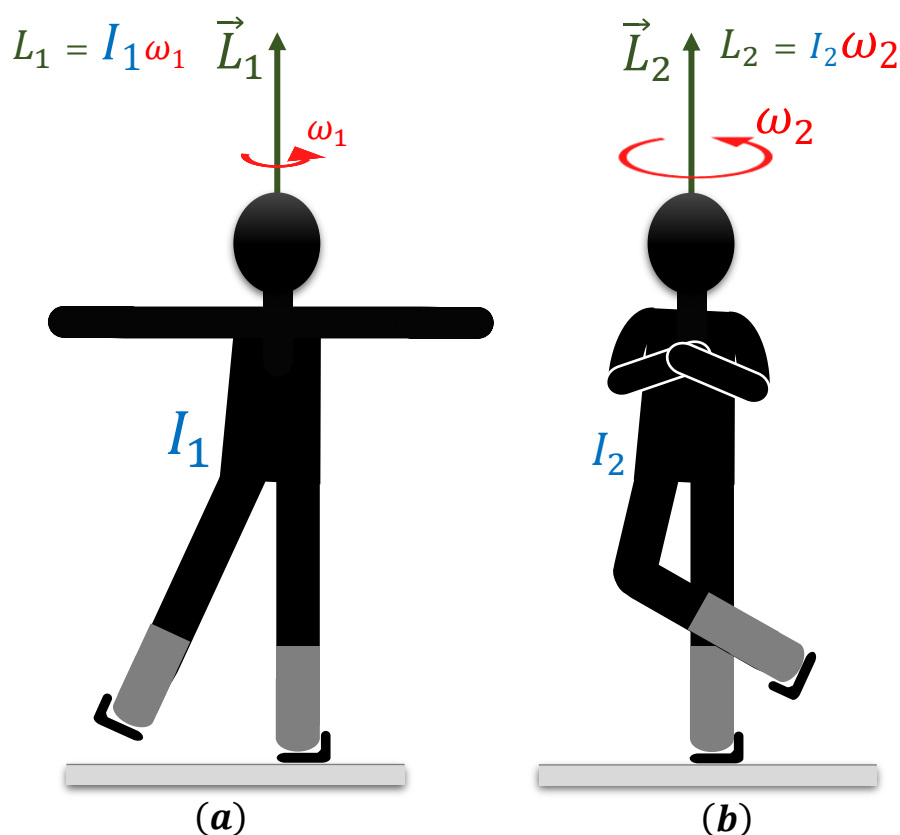
Figura 45 - Patinador de gelo girando em torno do seu eixo vertical
