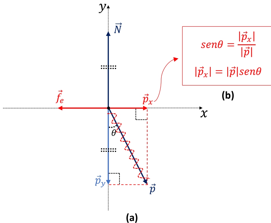
Figura 39 - Representação das forças que agem no corpo redondo da Fig. (38)
