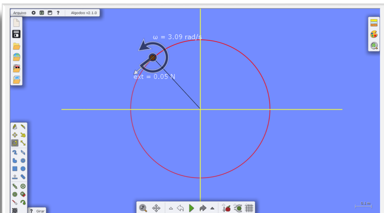
Figura 6.03: Captura de tela do software Algodoo : corpo de massa m preso à extremidade de uma barra fina de massa desprezível, submetido a uma força tangencial de 0,05 N e com velocidade angular de 3,09 rad/s. Fonte: os autores.
