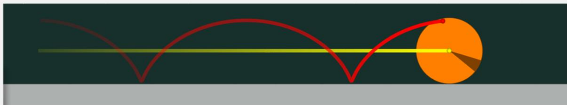
Figura 7.08: Recorte de captura de tela do software Algodoo : trajetórias de dois pontos distintos em um movimento de rolamento. Fonte: os autores.
