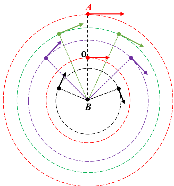
Figura 35 - Movimento de rolagem como uma rotação pura
