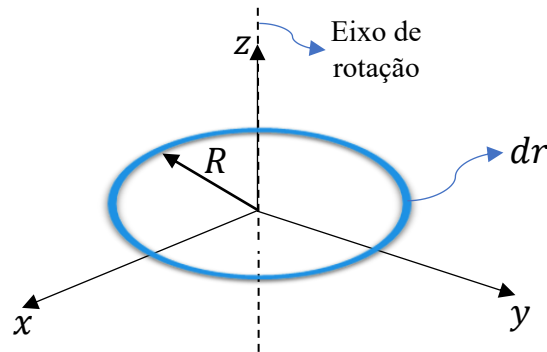
Figura 20 - Anel fino com eixo central de rotação
