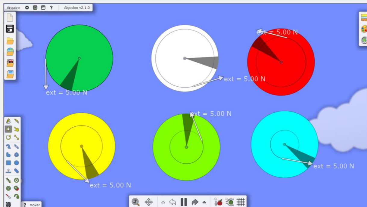
Figura 5.02: Captura de tela do software Algodoo: torques diferentes para forças iguais aplicadas em corpos idênticos.
