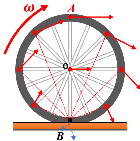
Figura 35 - Movimento de rolagem como uma rotação pura
