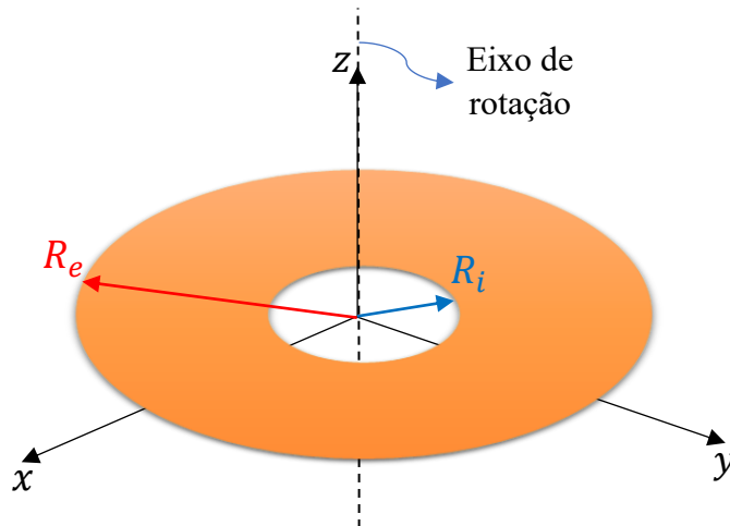
Figura 17 - Coroa circular com eixo de rotação no seu centro de
