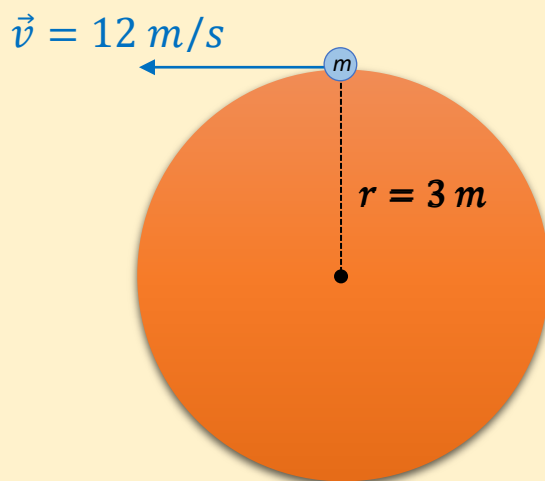
Figura 11.05: Exercício Resolvido 11.01: Momento angular de uma partícula de massa m em movimento circular uniforme.
