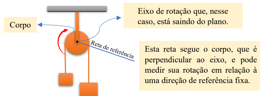
Figura 1 - Polia em movimento de rotação em relação a um eixo fixo
