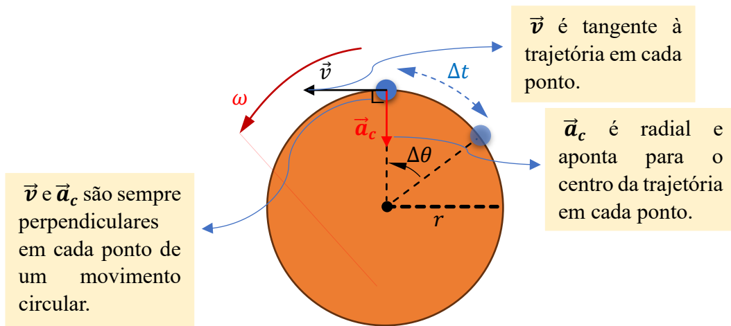
Figura 6 - Disco rígido com uma partícula em MCU
