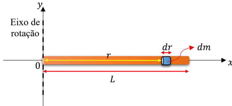
Figura 16 - Barra fina homogênea com eixo de rotação em uma de suas extremidades
