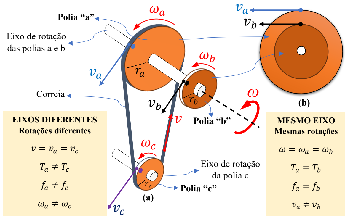
Figura 8 - Transmissão de rotação entre polias
