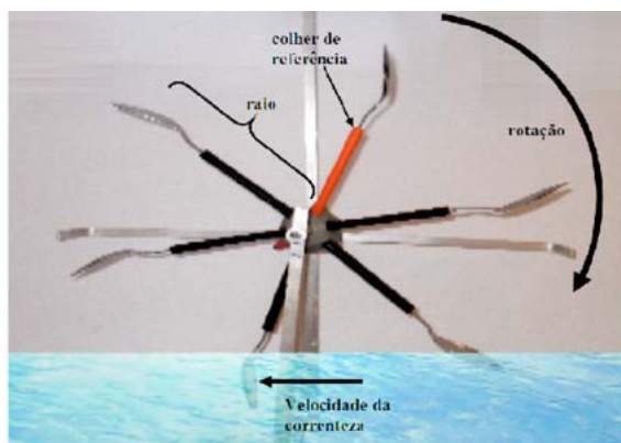
Figura 2 – Variáveis analisadas no funcionamento do molinete eletroindutivo.
