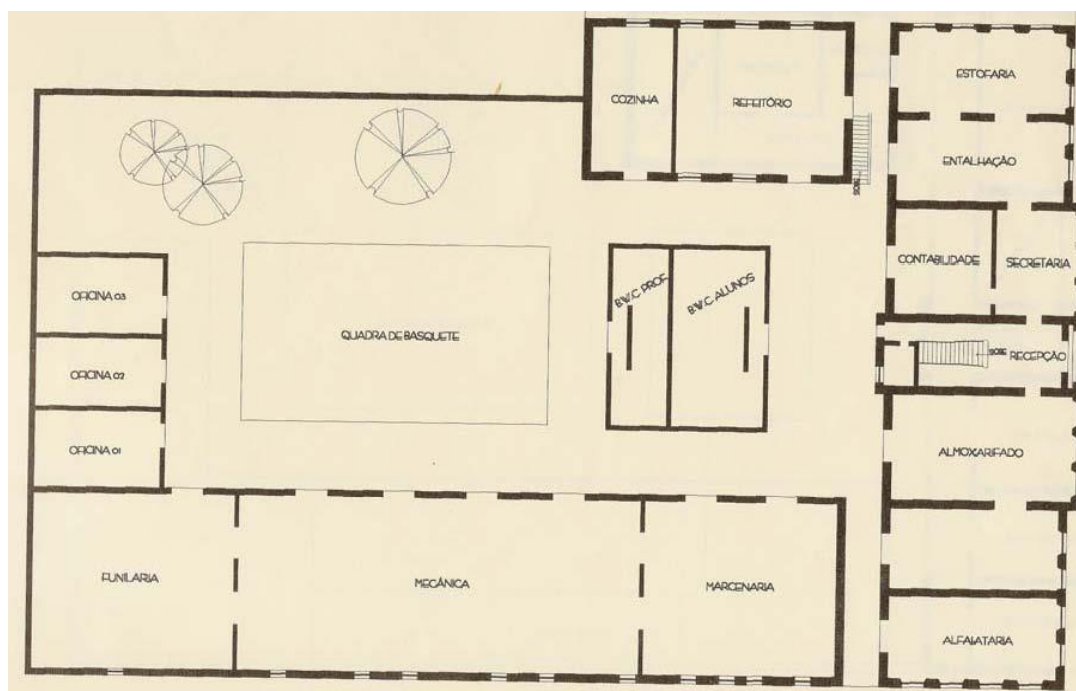
Figura 1 – Planta baixa do pavimento térreo da EIN (1940)
