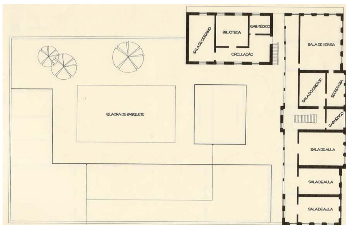
Figura 2 – Planta baixa do pavimento superior da EIN (1940).
